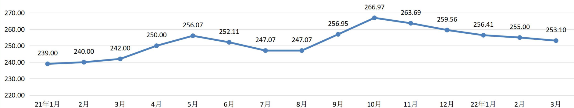
预应力高强混凝土管桩 AB型 PHC \Phi 500 \times 125 单位:元/m
